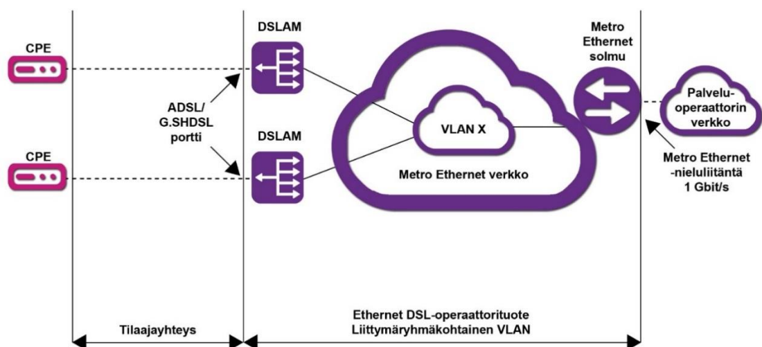
Kuva 3: Ethernet DSL-operaattorituote, liittymäryhmäkohtainen VLAN ja tilaajayhteys
