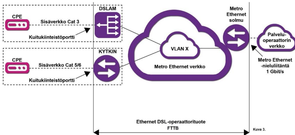
Kuva 1: DSL-operaattorituote Kuitukiinteistöportti
