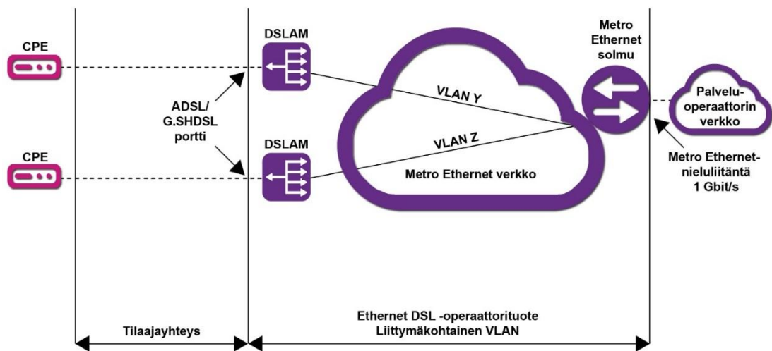
Kuva 4: Ethernet DSL-operaattorituote, liittymäkohtainen VLAN ja tilaajayhteys
